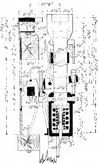
Fig. 2350. Longitudinal Section.
